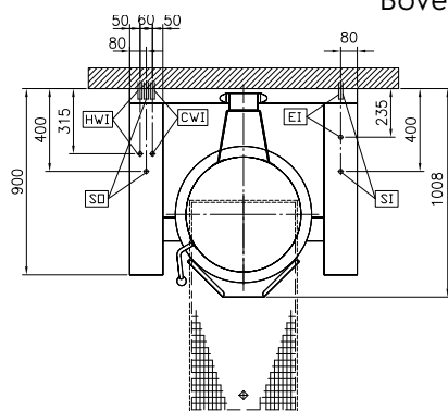
Boven aanzicht
